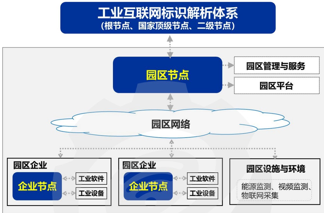
图3 工业互联网园区标识节点示意图
