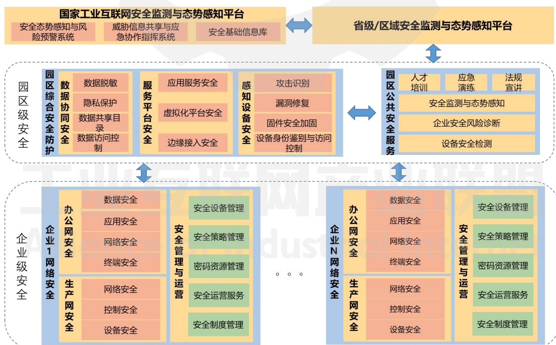
图 6 工业互联网园区安全架构
